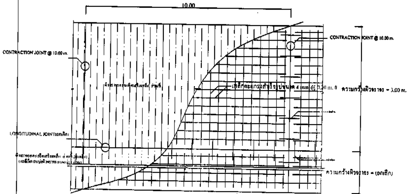
แผนทั่วไปของคอนกรีตเสริมเหล็ก NOT TO SCALE
