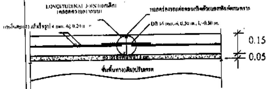
แบบขยาย LONGITUDINAL JOINT (ขกลึก)
