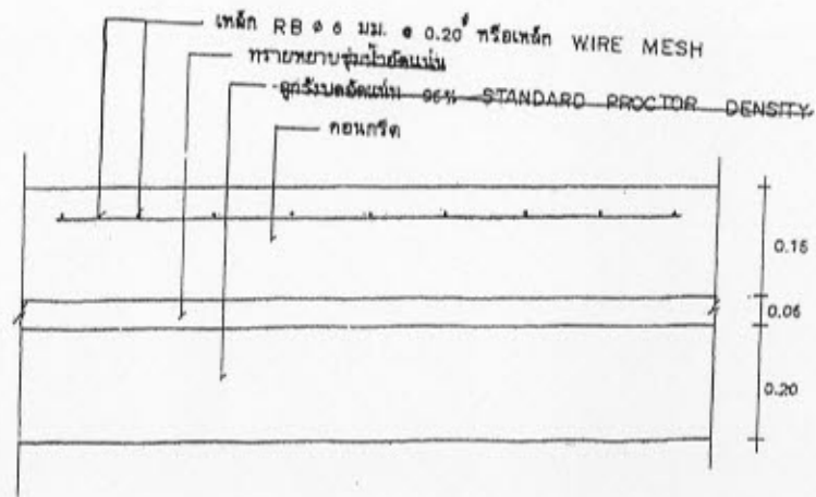
รายละเอียดความหนาแน่นคอนกรีตบริเวณเหล็ก NOT TO SCALE
