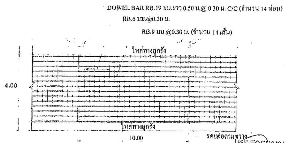
รูปแปลนถนนผิวจราจรคอนกรีต
