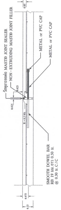
ขยายรอยต่อ EXPANSION JOINT (ทุกระยะ 100 เมตร)
