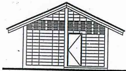
รูปด้านหลัง มาตราส่วน 1:100
