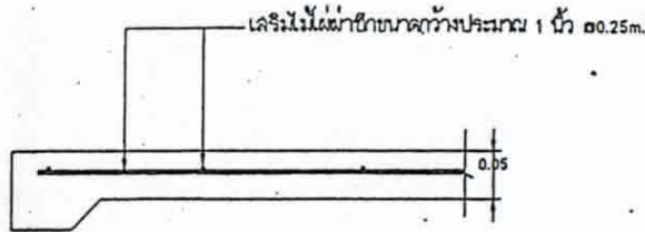
รูปตัด GS มาตราส่วน 1:20
