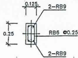
รูปตัด GB1 มาตราส่วน 1:20
