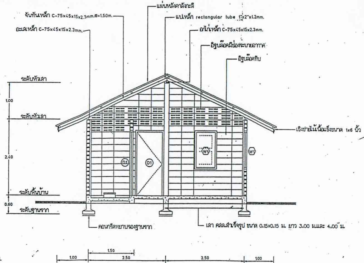
รูปตัด A - A SCALE 1:50
