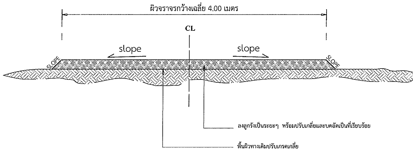
รูปตัดขวางถนนลูกรัง 1:35
