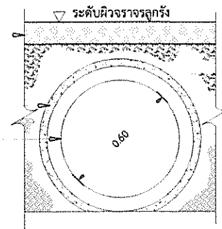
รูปตัดขวางท่อระบายน้ำ 1:35
