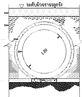
รูปตัดขวางท่อระบายน้ำ 1:35
