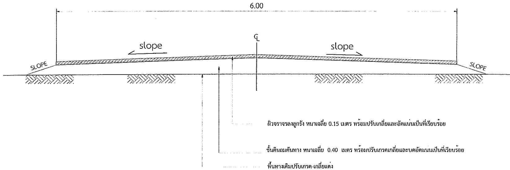
รูปตัดขวางถนนลูกริ่ง 1:35
