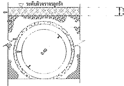
รูปตัดขวางท่อระบายน้ำ 1:15
