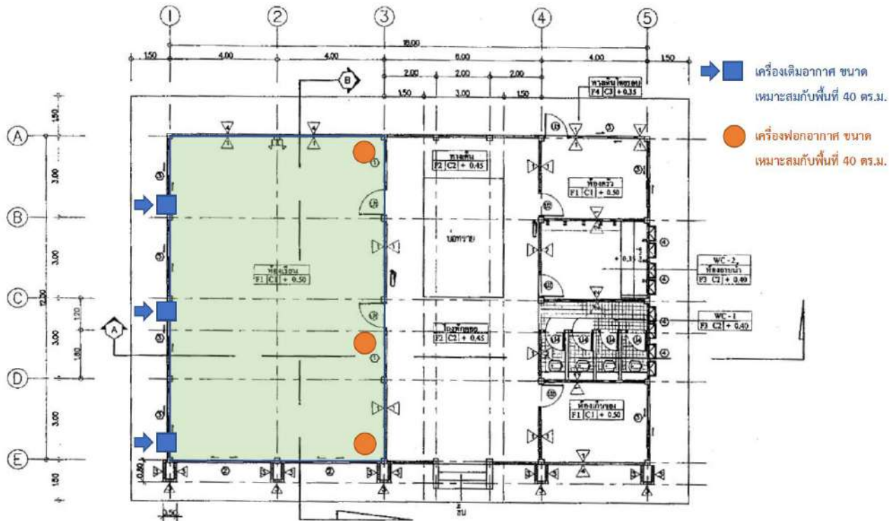
แบบแปลนมาตรฐานสำหรับการพัฒนาห้องปลอดฝุ่น ในศูนย์พัฒนาเด็กเล็ก ศพด. 1 ขนาดไม่เกิน 50 คน
