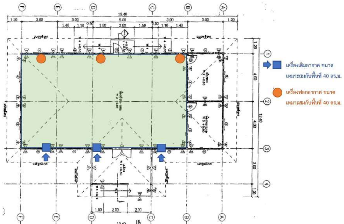
แบบแปลนมาตรฐานสำหรับการพัฒนาห้องปลอดฝุ่น ในศูนย์พัฒนาเด็กเล็ก ศพด. 2 ขนาด 51-80 คน
