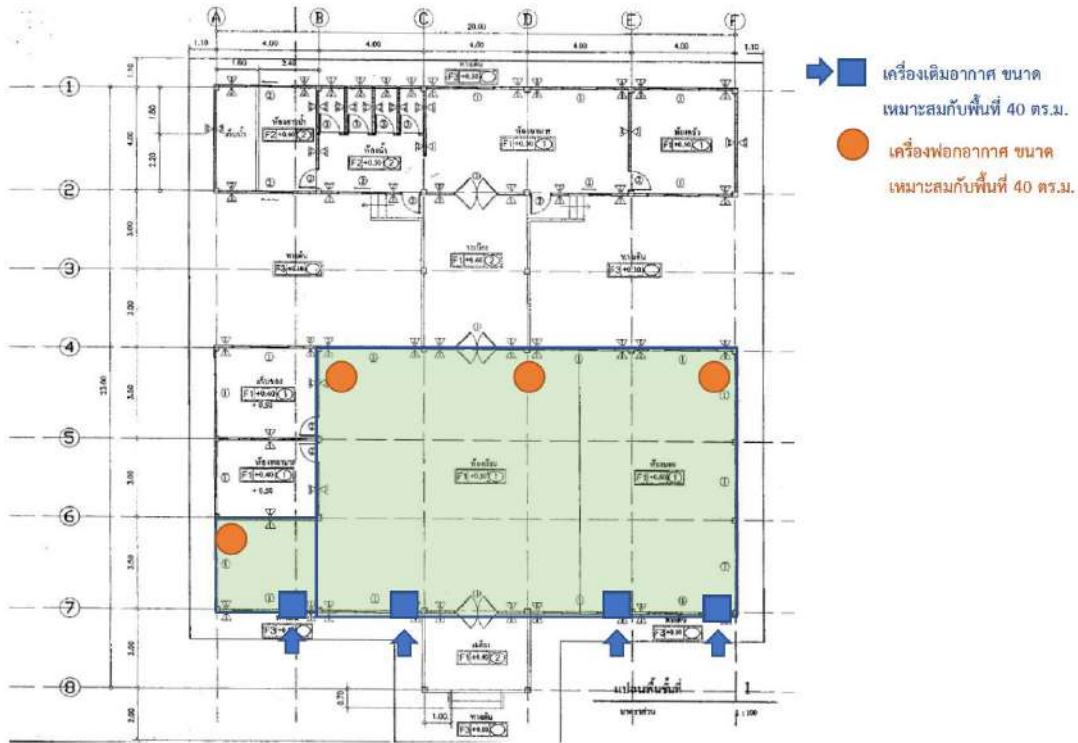
แบบแปลนมาตรฐานสำหรับการพัฒนาห้องปลอดฝุ่น ในศูนย์พัฒนาเด็กเล็ก ศพด. 3 ขนาด 81-100 คน
