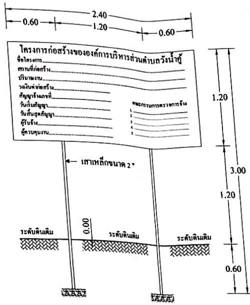
แบบป้ายโครงการ NOT TO SCALE
