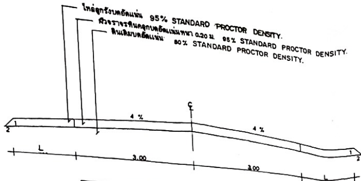
รูปตัดถนนผิวจราจรหินคลุกหนา 0.20 1:50
