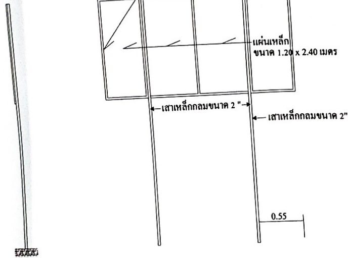
รูปด้านหลัง NOT TO SCALE
