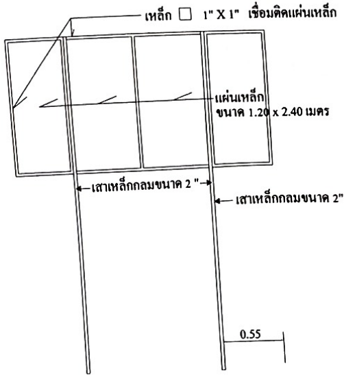
รูปด้านหลัง NOT TO SCALE
